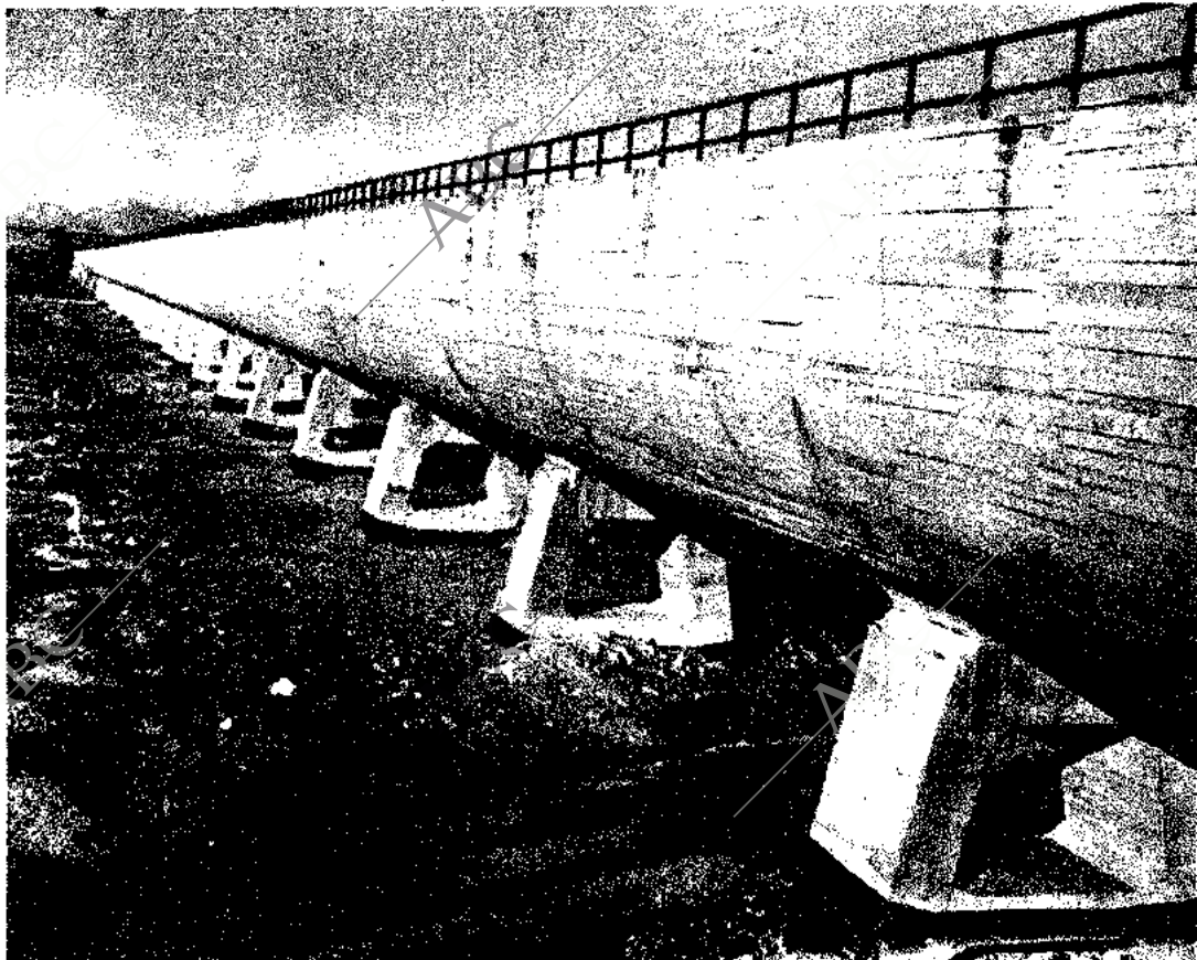
Acueducto de Tardienta, en el sistema de riegos de Los Monegros.
